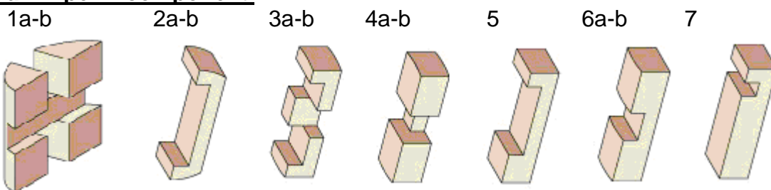
Figura 1 – pezzi componenti
